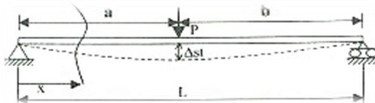
Gambar 1. Mekanisme Konstruksi Tumpuan Sederhana
