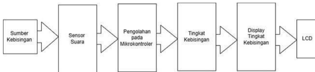
Gambar 1. Diagram Blok Sistem Tingkat Kebisingan
