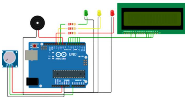
Gambar 3. Skema Rangkaian
